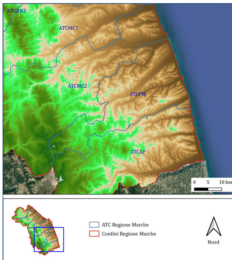
Figura 17 - Inquadramento dell'ATC Fermo su DTM.
